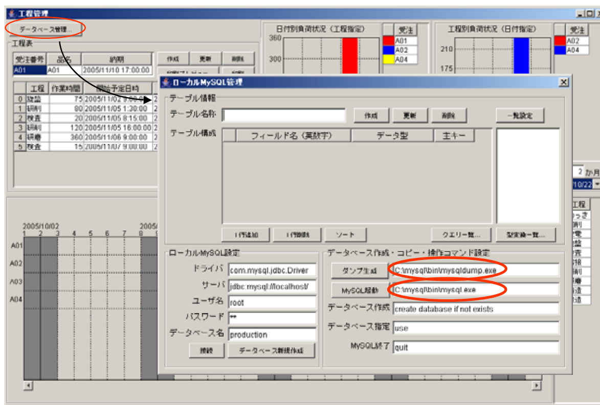
図 22 MySQL ダンプ生成コマンドと起動コマンドの指定
