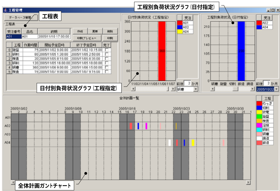
図 16 工程管理システム簡易版概観（再掲）
