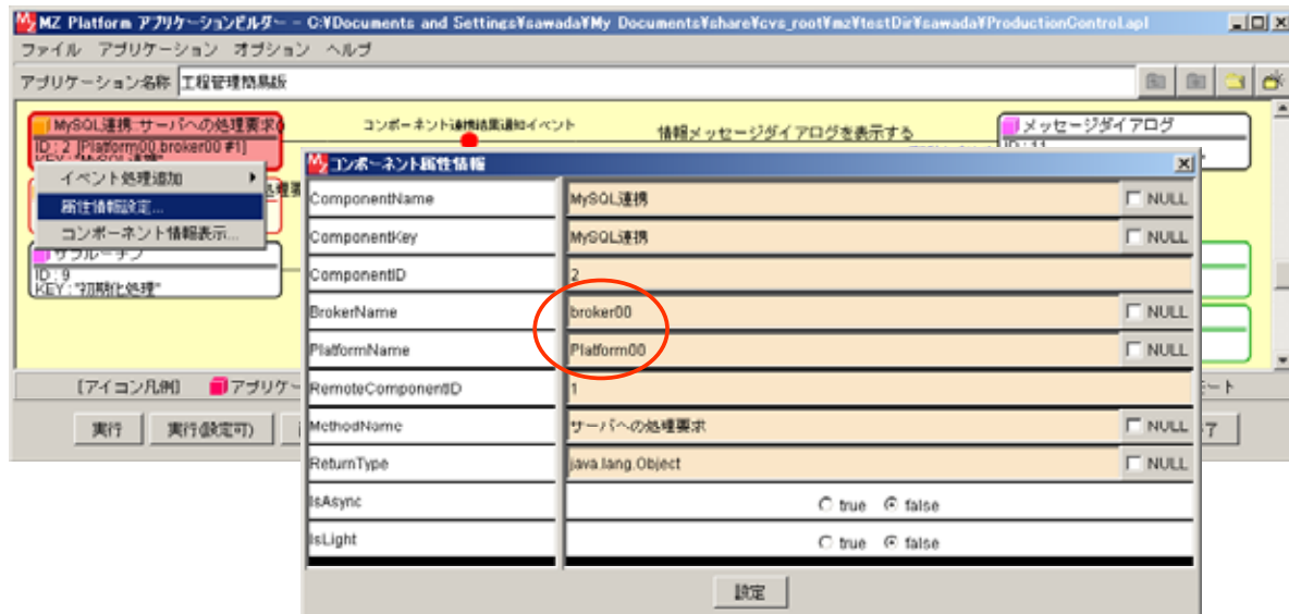
図 23 データ連携プラットフォーム設定変更（サーバ）
