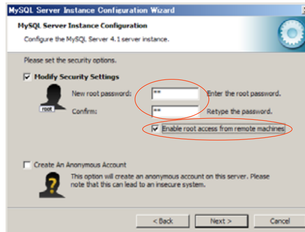
図 8 セキュリティ設定画面 (MySQL 4.1.14)
