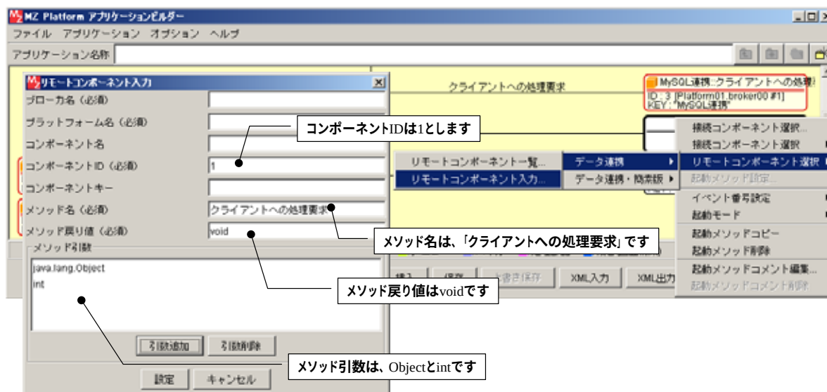
図 25 クライアントの追加
