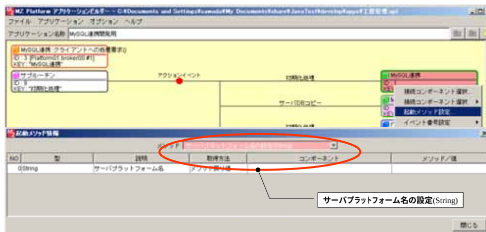
図 24 サーバプラットフォーム名の設定
