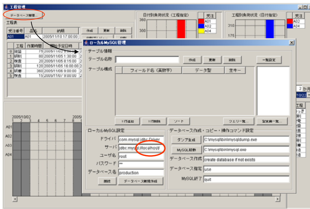
図 21 ローカル MySQL 管理ウィンドウの起動
