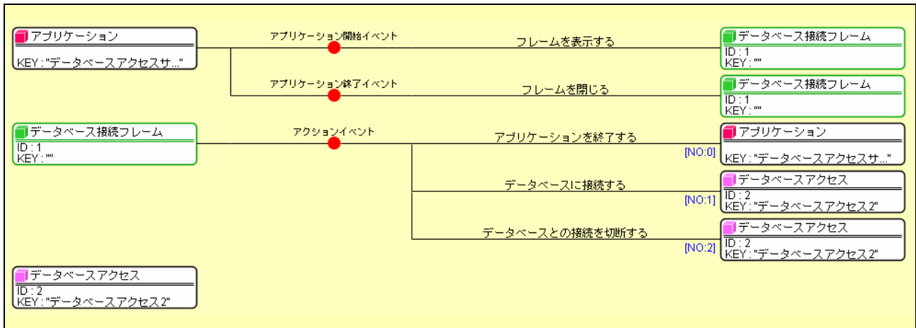
図 5 データベースアクセスアプリケーションのコンポーネント接続関係 (その1)
