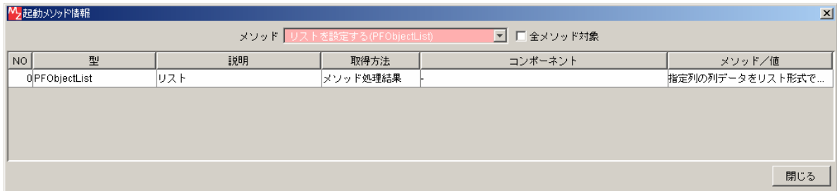
接続先コンポーネント（[リスト格納変数] コンポーネント②）の起動メソッドの設定画面
