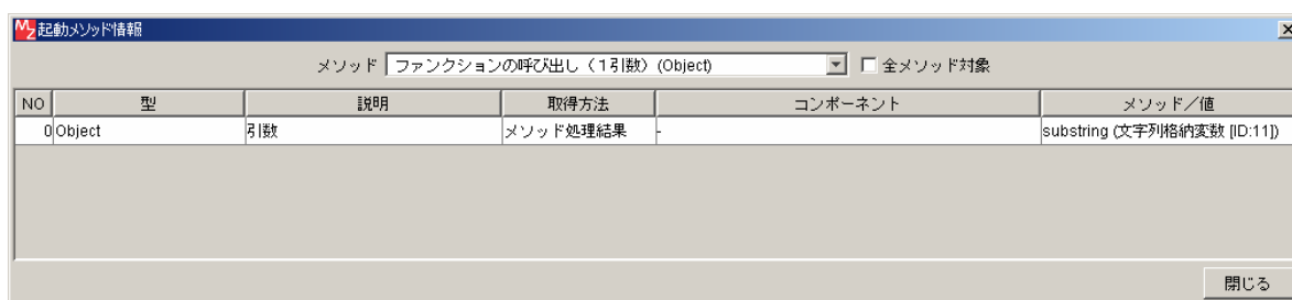
接続先コンポーネント ([ファンクション] コンポーネント②) の起動メソッドの設定画面
