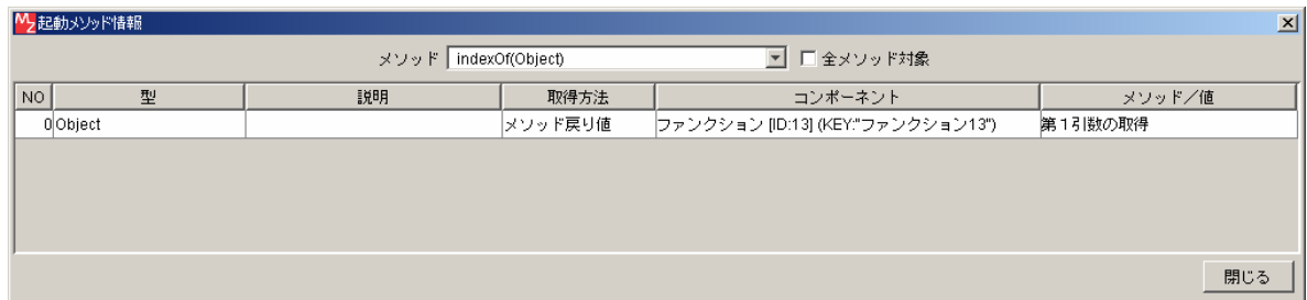
接続先コンポーネント（[リスト格納変数] コンポーネント③）の起動メソッドの設定画面
