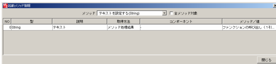
接続先コンポーネント ([テキストフィールド] コンポーネント③) の起動メソッドの設定画面
