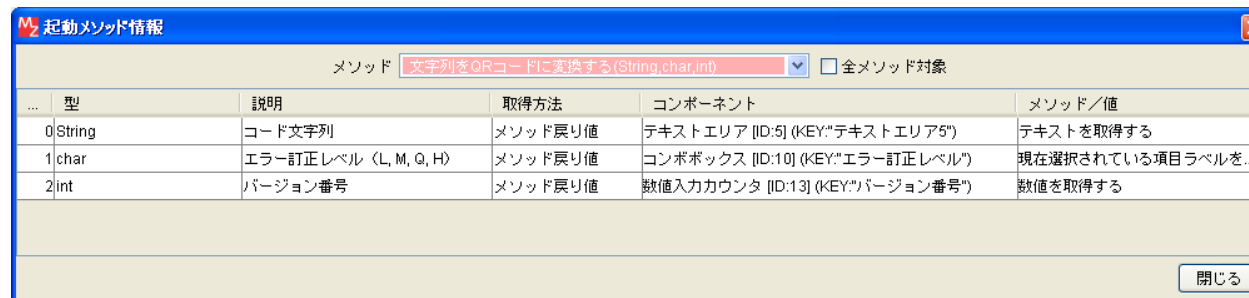
図 6 「文字列をQRコードに変換する(String,char,int)」メソッド
