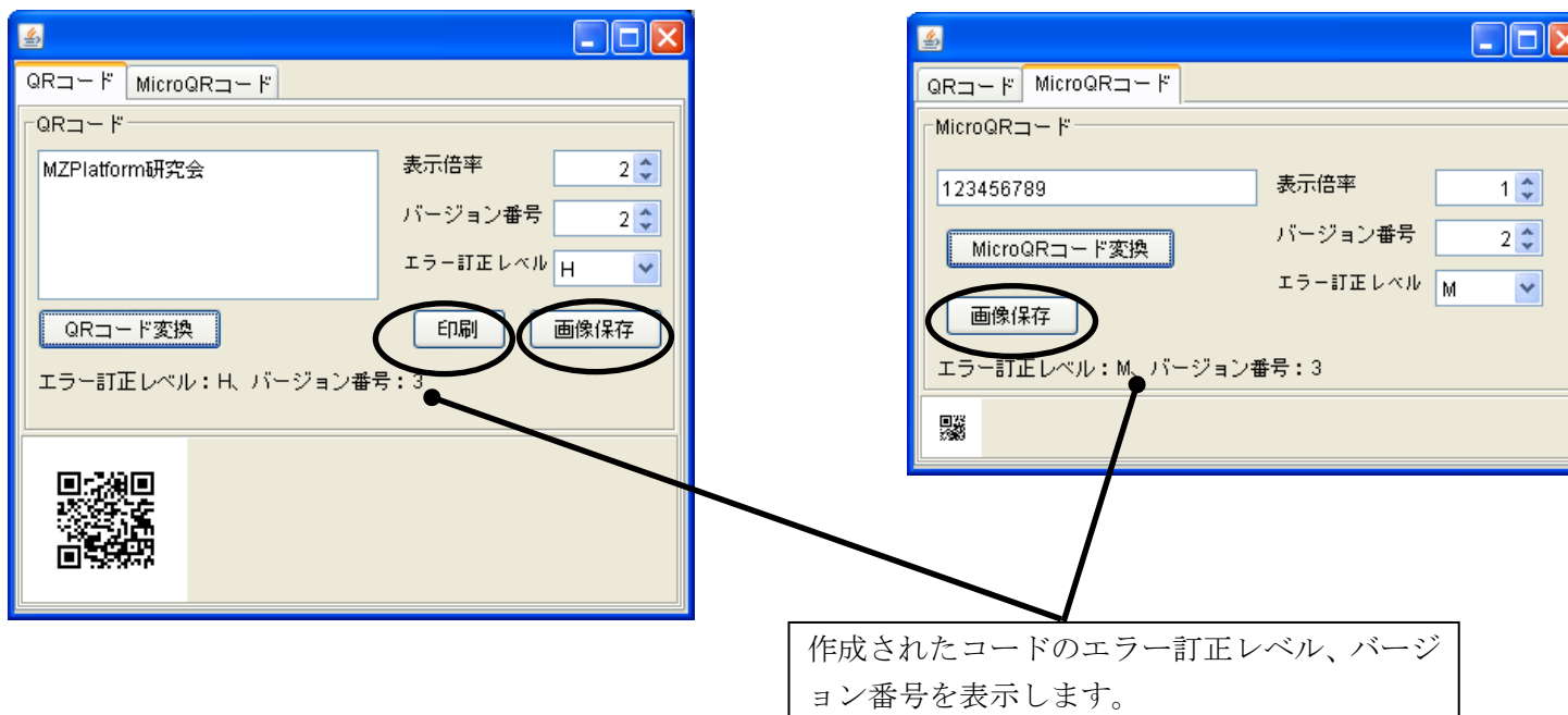
図 2 QRコードの表示
