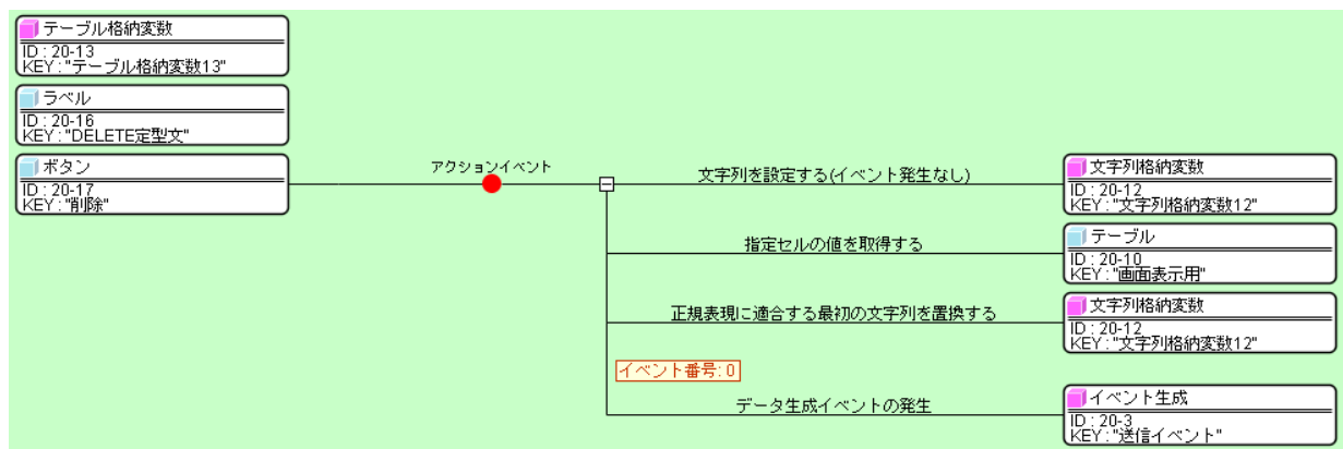
図 69 削除機能の作成(コンポーネント接続関係)
