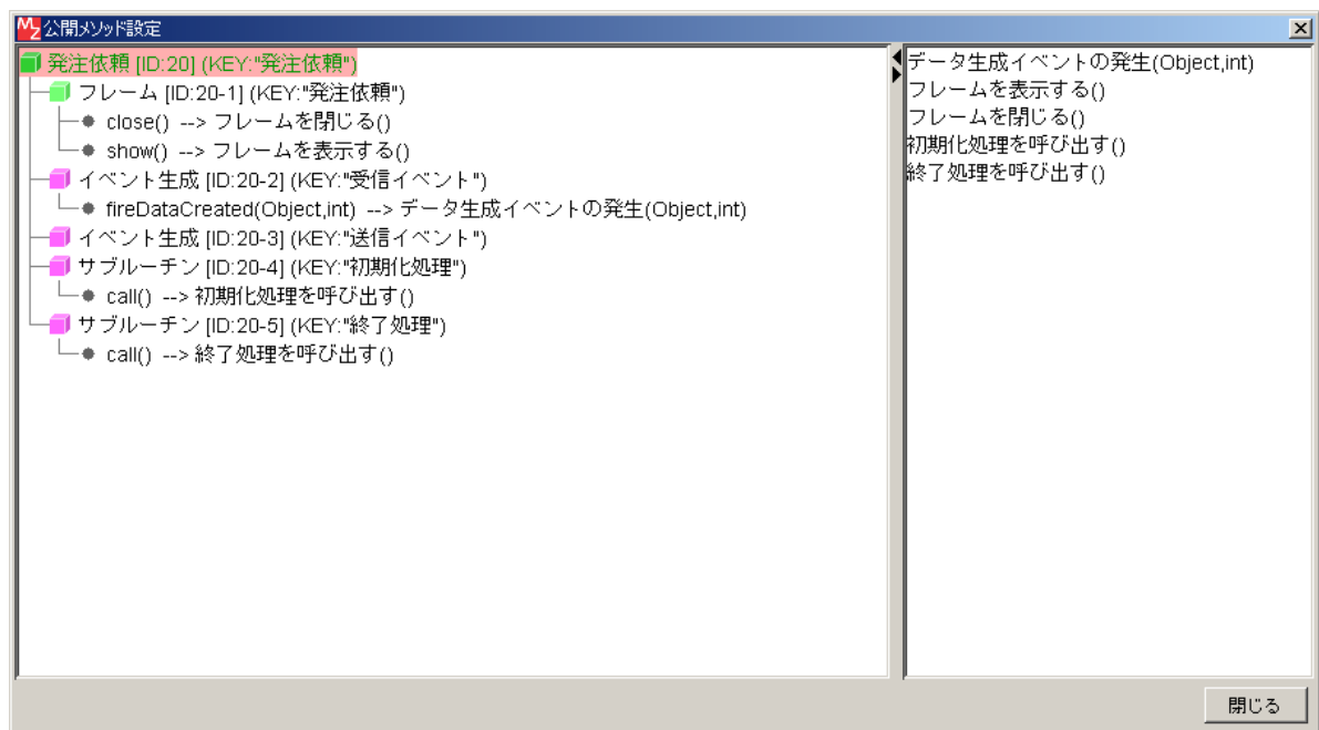
図 53 公開メソッドの設定コンポーネント接続の初期設定
