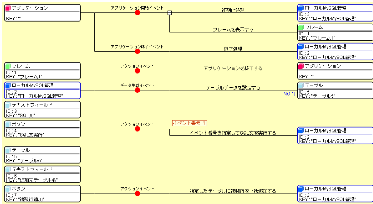
図 30 複数行一括追加機能の追加 (コンポーネント接続関係)
