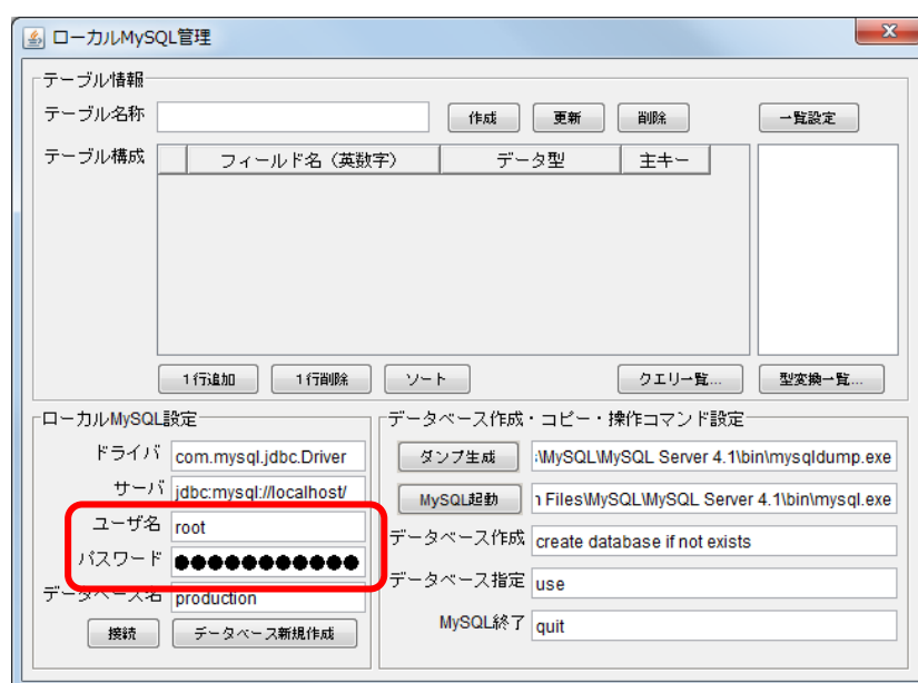
図 13 MySQL のユーザ名とパスワードの設定
