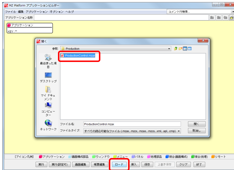
図 10 工程管理システム簡易版のロード
