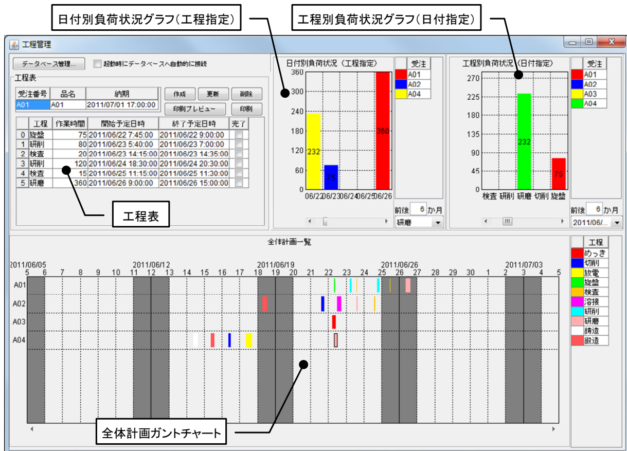
図 17 工程管理システム簡易版概観 (再掲)
