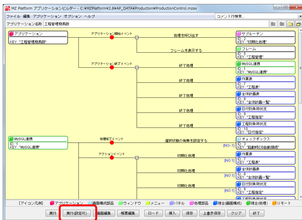
図 11 工程管理システム簡易版の起動
