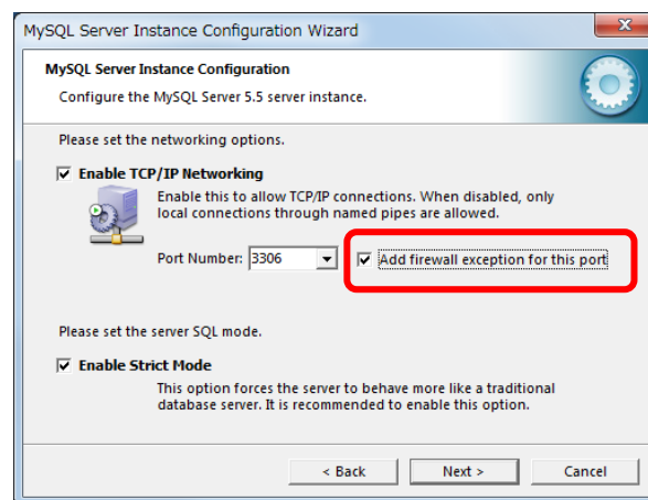
図 8 ネットワークオプション設定画面
