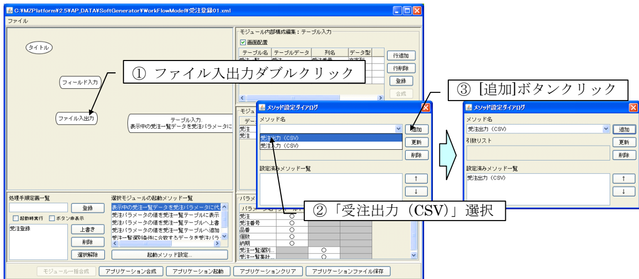
図 46 ファイル入出力モジュールの起動メソッド設定（CSV 出力用）
