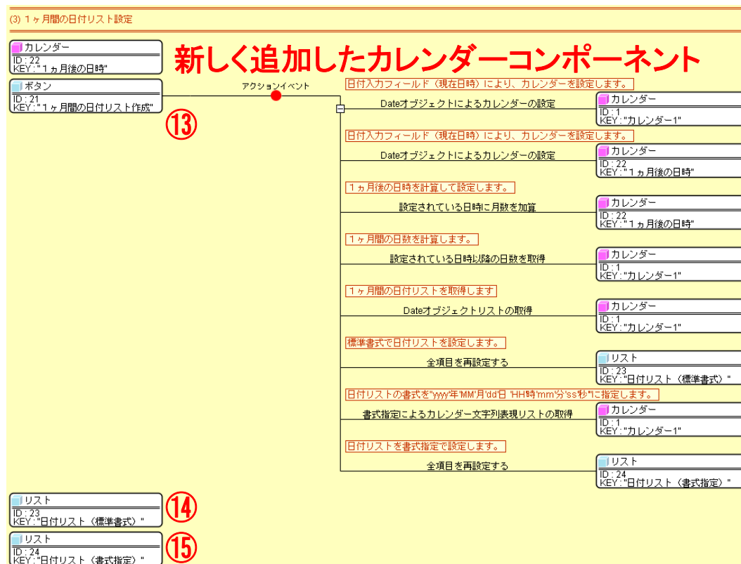
図 10 1ヶ月間の日付リスト設定に関わるコンポーネント接続図
