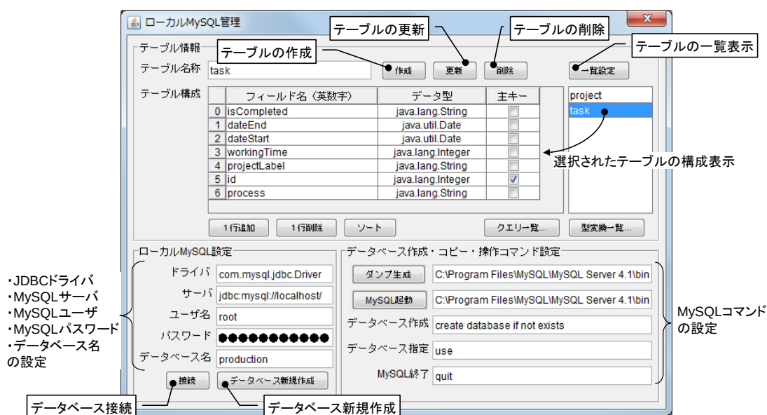
図 27 ローカル MySQL 管理複合コンポーネント
