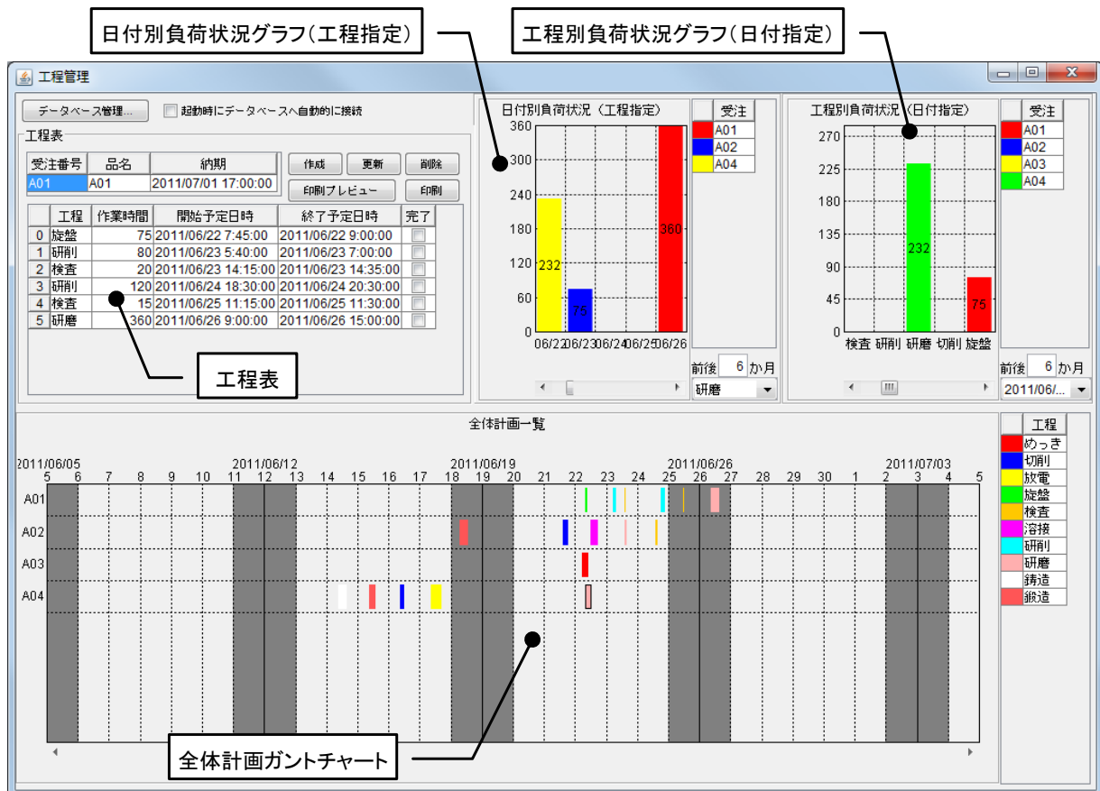
図 21 工程管理システム簡易版概観(再掲)
