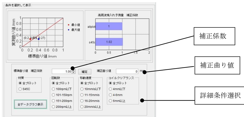
図9 高周波焼入れ変形予測テンプレート C 工程設計部
