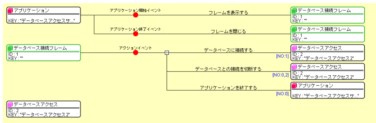
図 5 データベースアクセスアプリケーションのコンポーネント接続関係（その 1）
