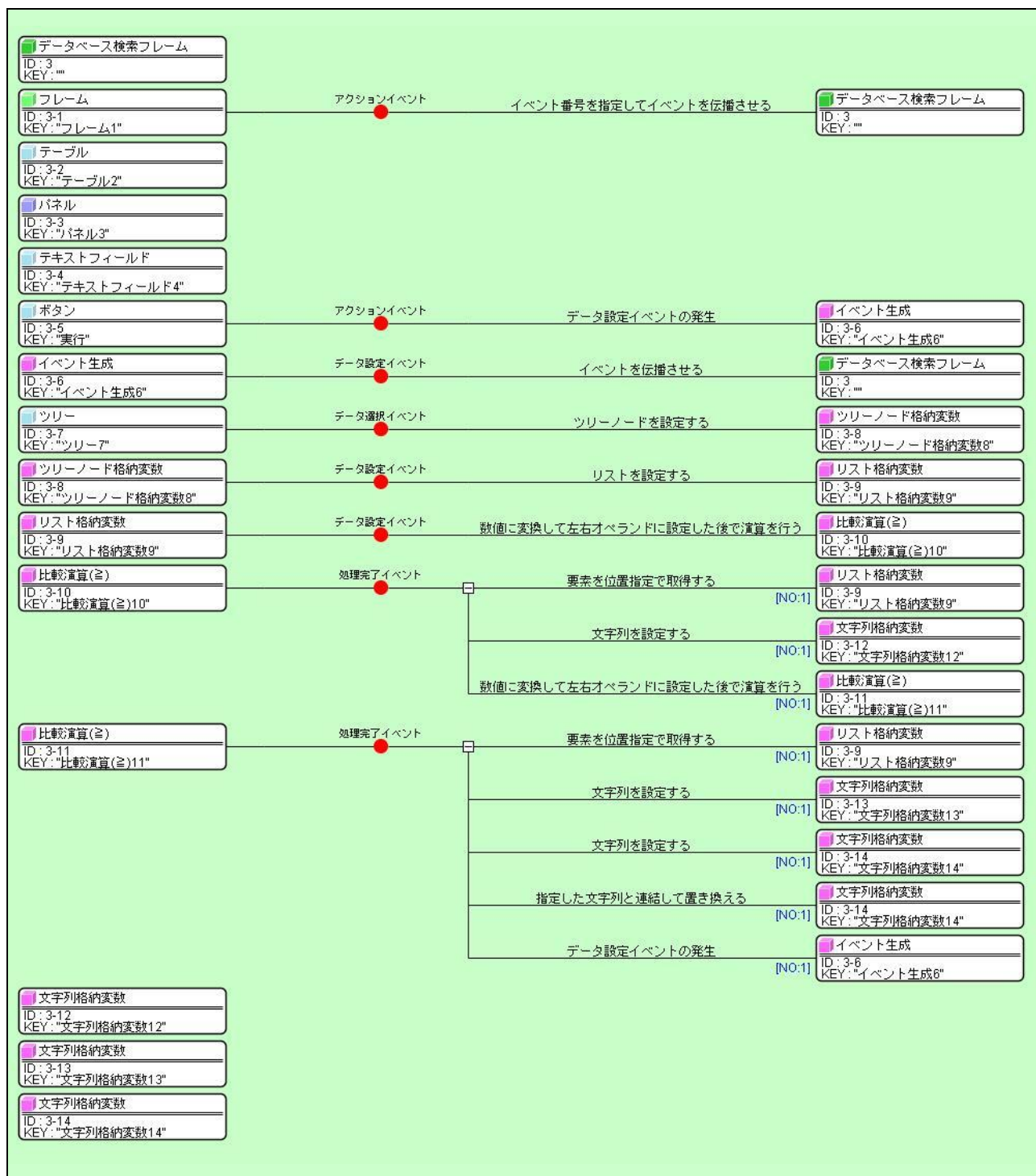
図 11 データベース検索フレームのコンポーネント接続関係（その2）
