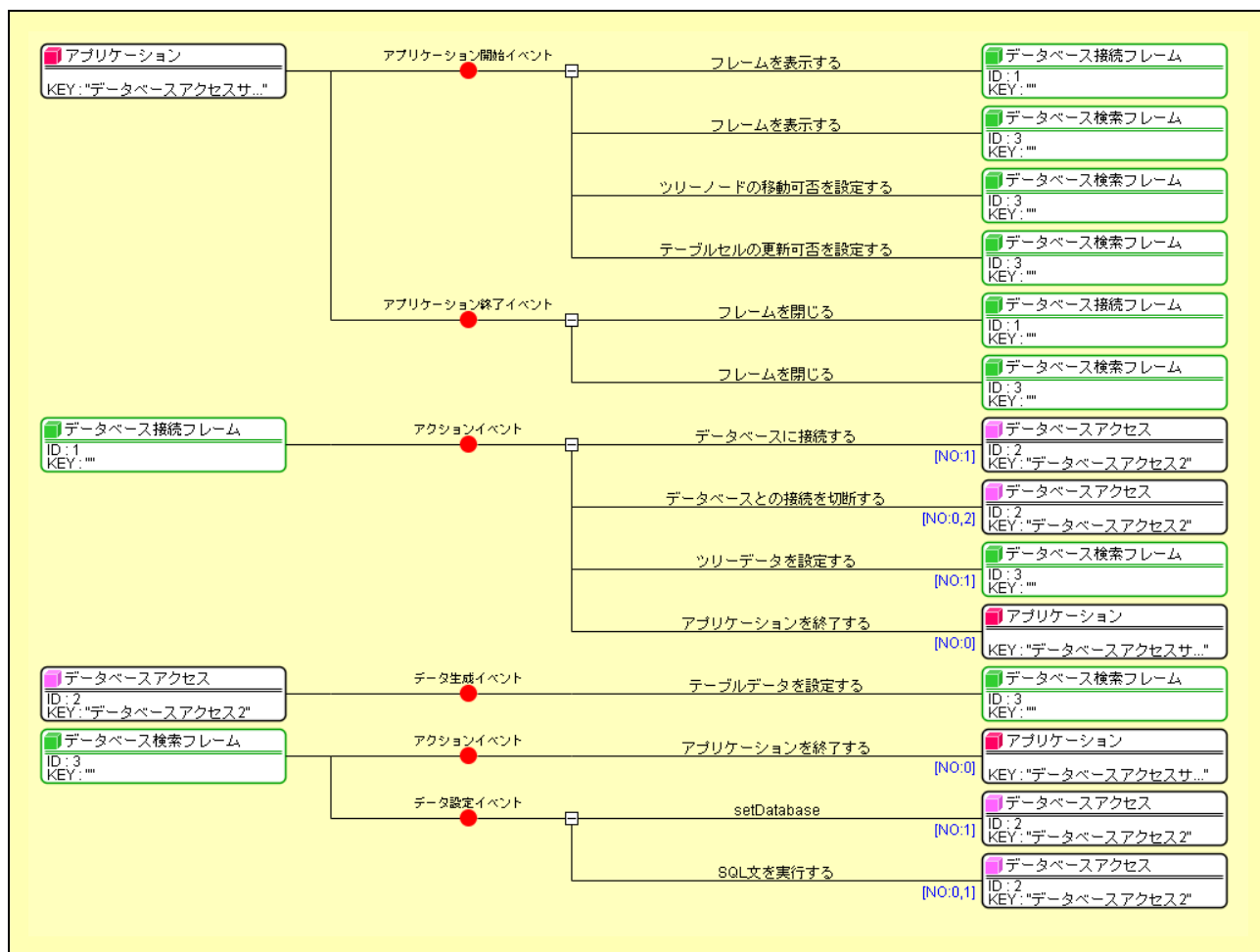
図 17 データベースアクセスアプリケーションのコンポーネント接続関係（その 5）
