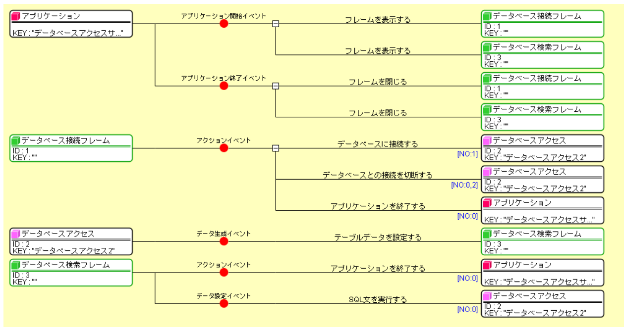
図 8 データベースアクセスアプリケーションのコンポーネント接続関係（その 2）
