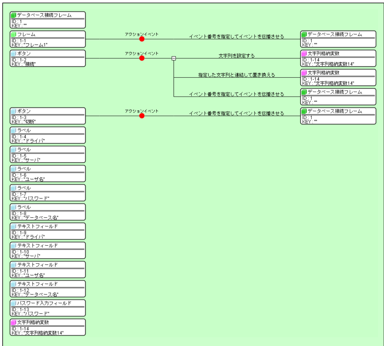
図 3 データベース接続フレームのコンポーネント接続関係
