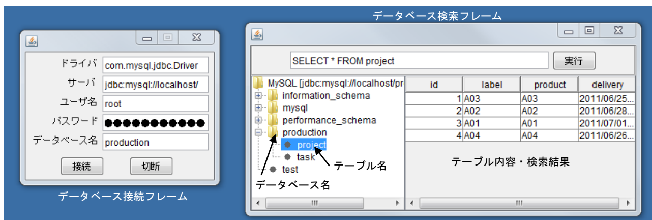
図 1 データベースアクセスアプリケーションの画面イメージ
