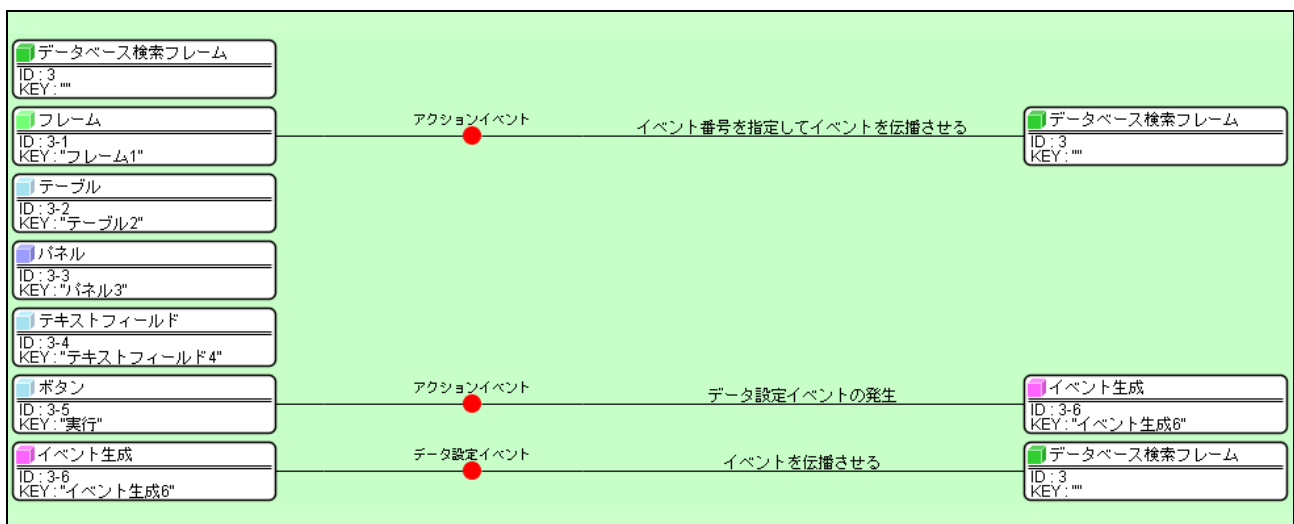
図 7 データベース検索フレームのコンポーネント接続関係 (その 1)
