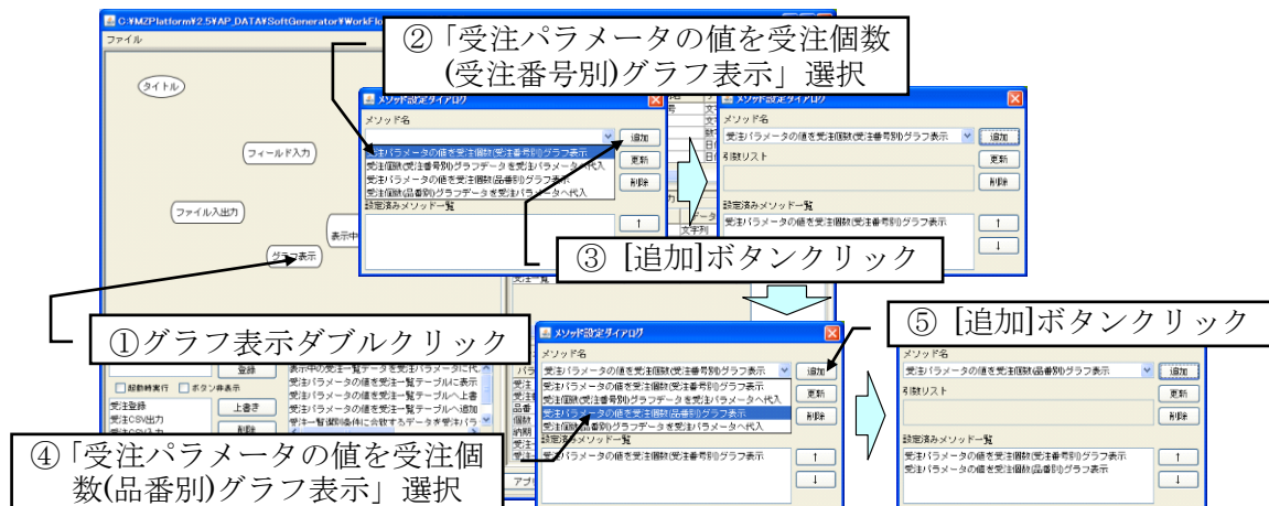
図 67 グラフ表示モジュールの起動メソッド設定（受注个数グラフ表示）
