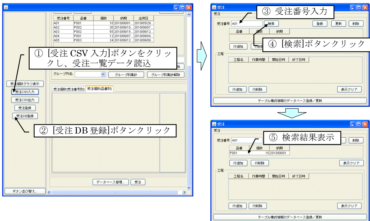
図 84 受注データの登録と検索
