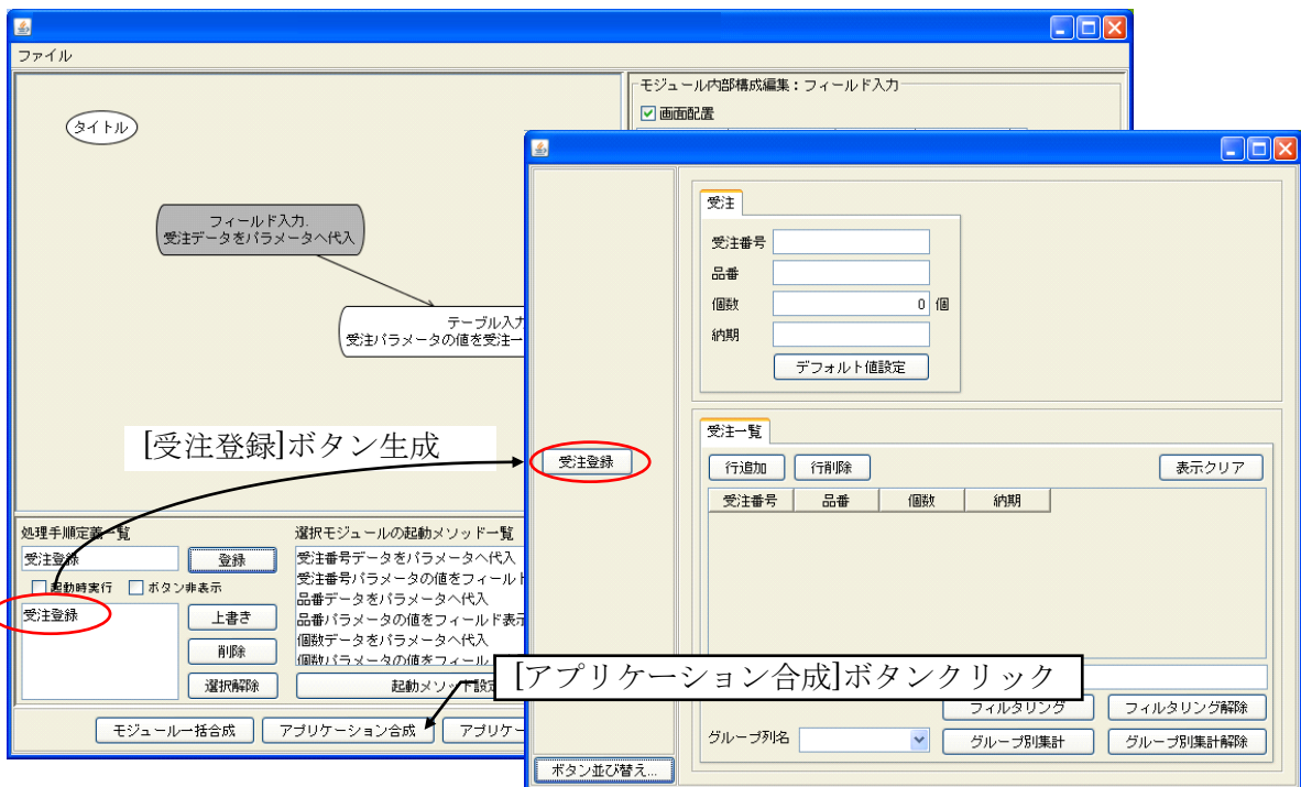
図 22 アプリケーションの合成
