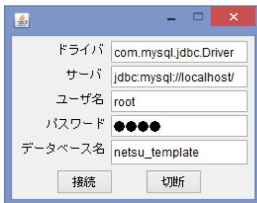
図 3 データベース接続設定画面
