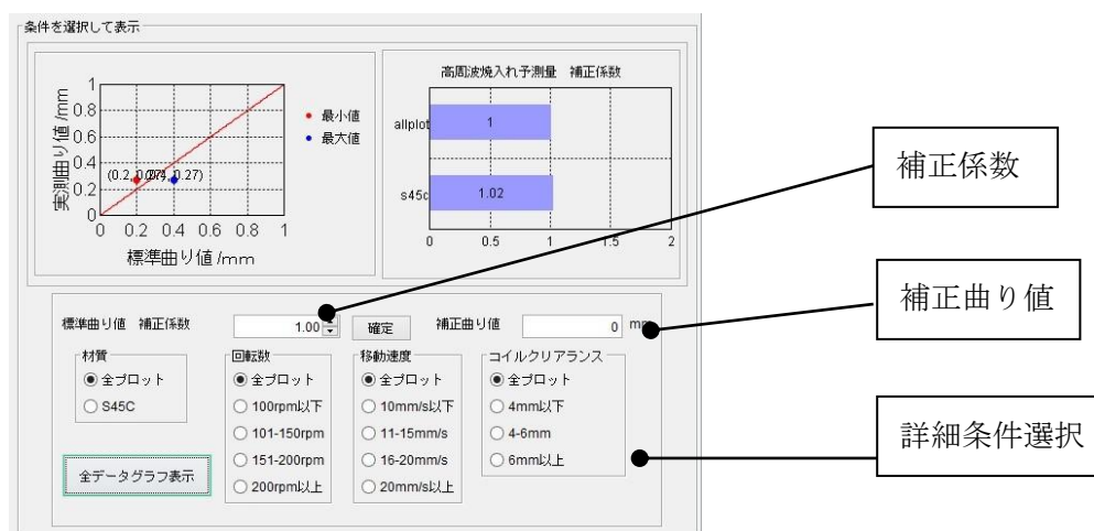
図 9 高周波焼入変形予測テンプレート C 工程設計部
